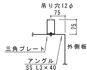
吊りネコ詳細
